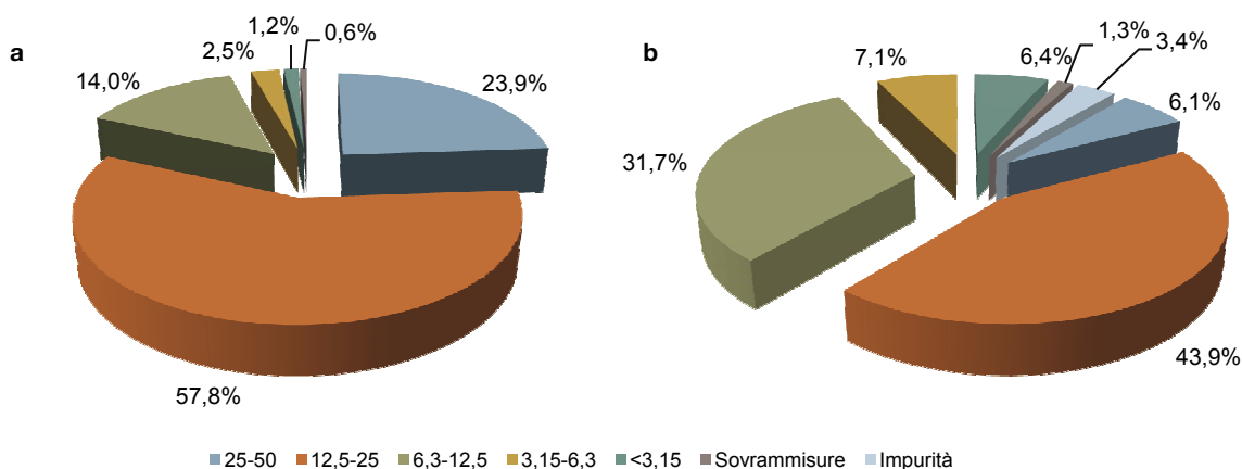
Grafico 1 - Analisi granulometrica relativa al cippato di pioppo ottenuto con (a) un rotore modificato CRA-ING e (b) rotore di serie (mod. da PARI et al. 2009).
