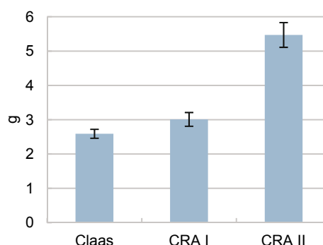
Grafico 2 - Peso medio delle scaglie di cippato della classe 16-45 mm prodotte dai 3 rotori.
