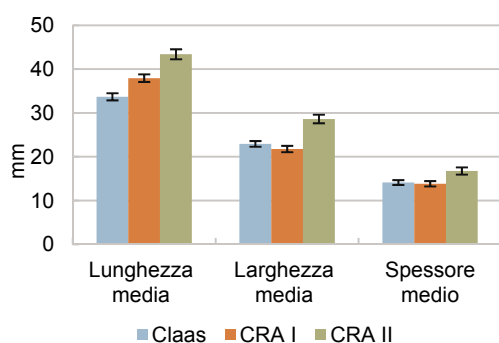
Grafico 1 - Lunghezza, larghezza e spessore medio ( \pm err. st.) delle scaglie di cippato della classe 16-45 mm prodotte dai 3 rotori.
